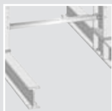
Longitudinal bracing
